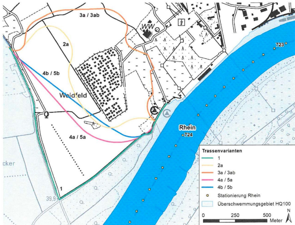
Lageplan Trassenvarianten
